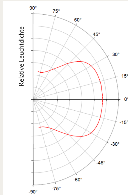
Abb. 2: Entblendungswirkung von PLEXIGLAS® Textures für Leuchten OA000 SL bei kantenbeleuchteten LED-Deckenleuchten
