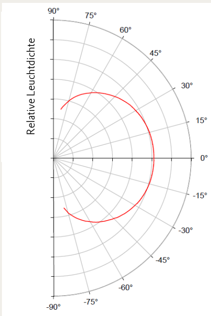
Abb. 1: Performance einer Standard-Lichtstreuerscheibe
